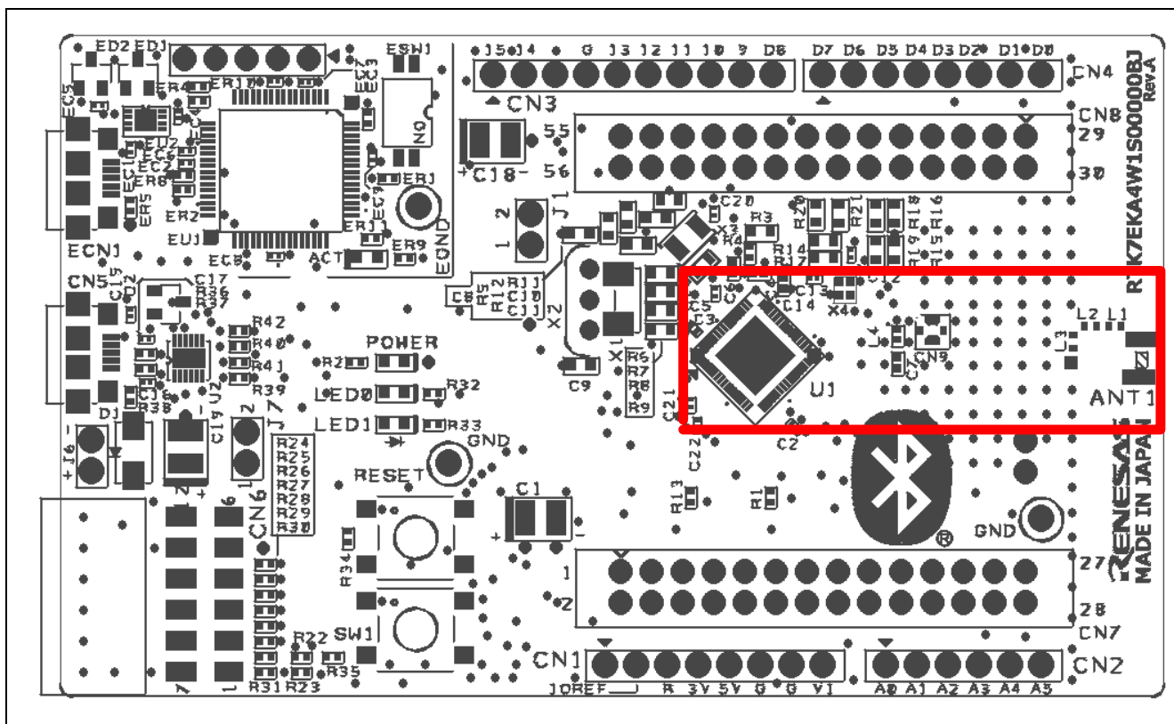
Figure 7. BLE Circuit
