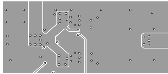
Inner Layer 2
