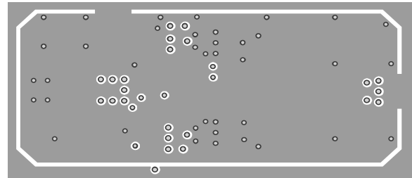
Inner Layer 1
