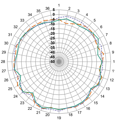
YZ-Plane Gain
